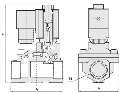
Рисунок 1. Эскиз
