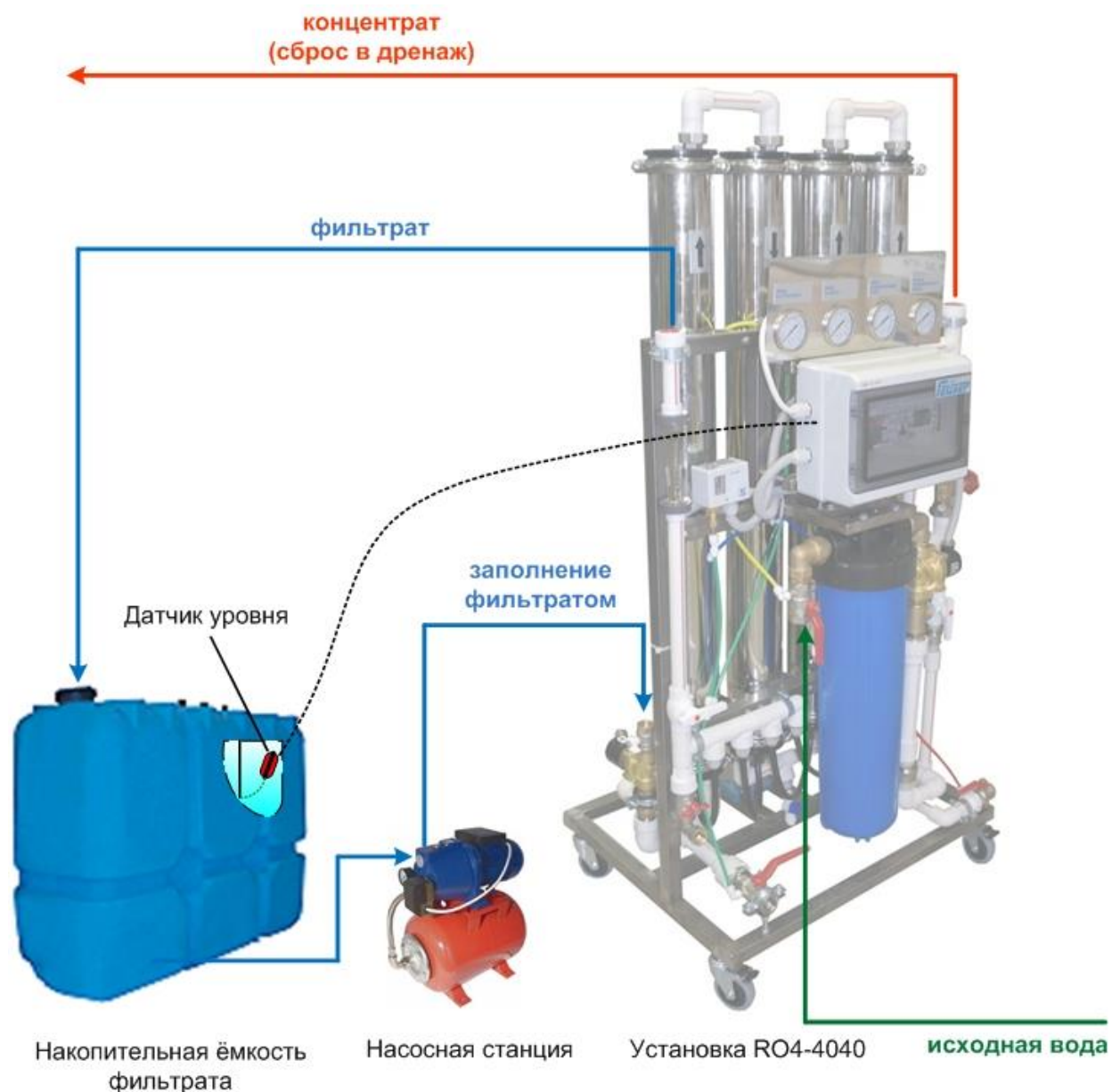
Рис. 5 Подключение трубопроводов к установке.
