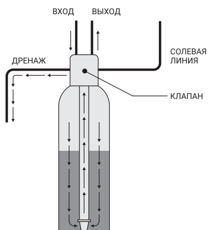
Прямая промывка – Этап 4
