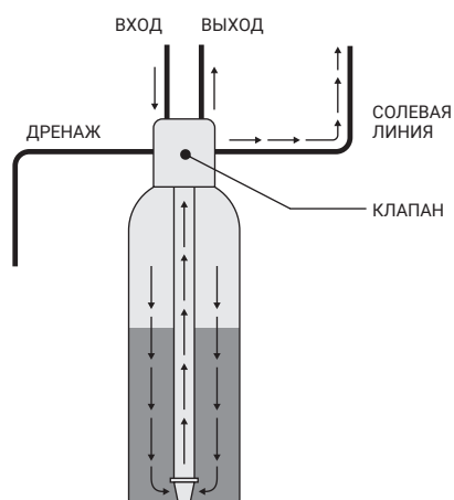
Заполнение бака-солеорастворителя – Этап 5
