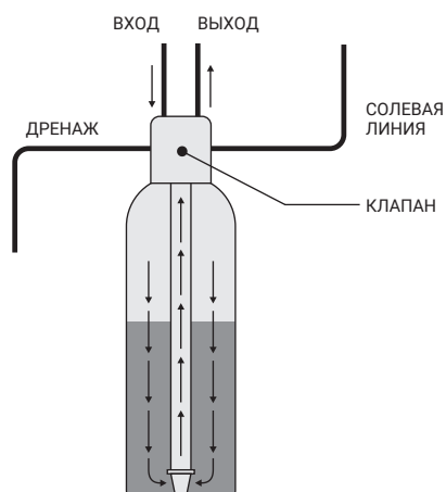
Пауза и задержка – Этап 1
