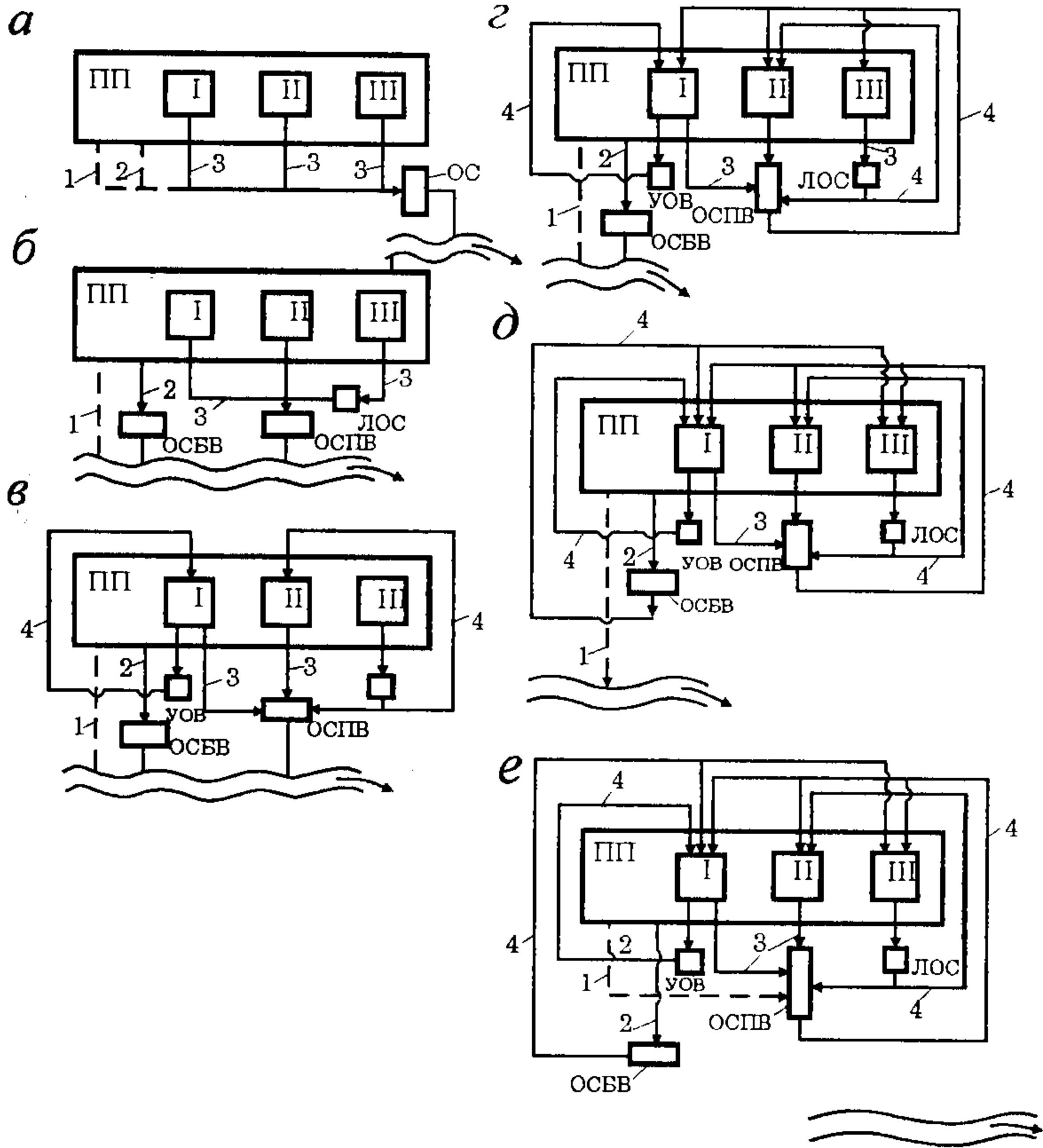
Рис. 1.7. Системы водоотведения промышленных предприятий:
