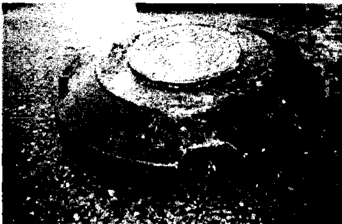
Рис. 6.10. Опорная железобетонная плита для горловин смотровых колодцев
