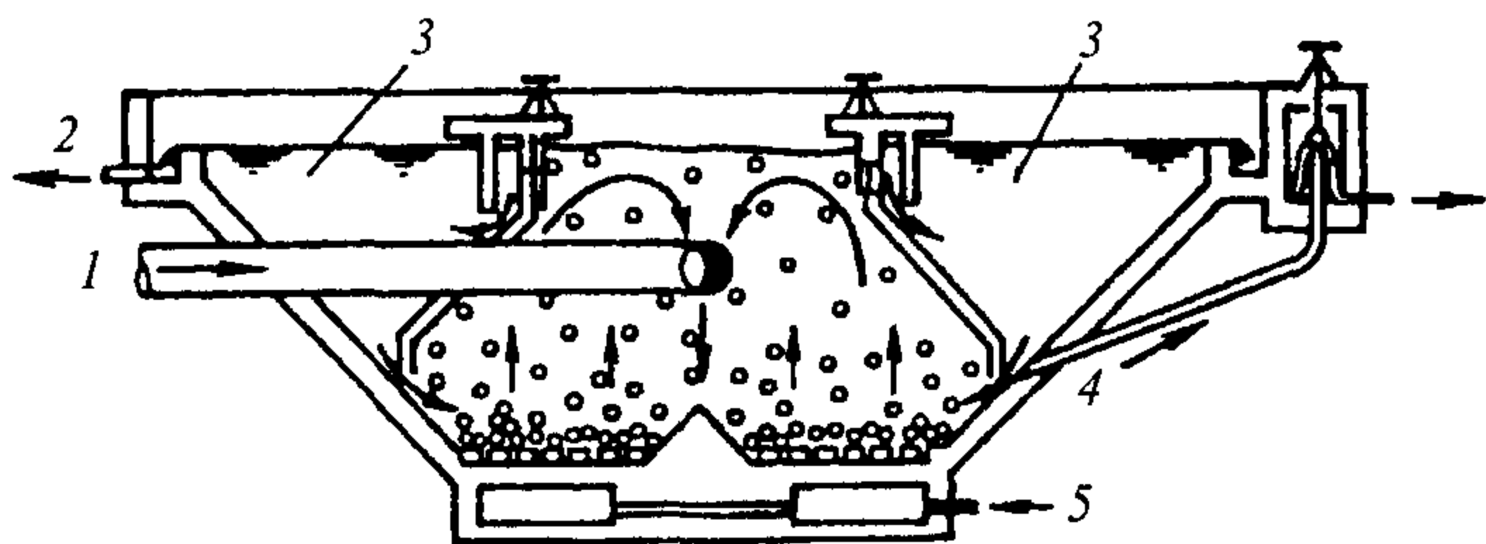
Рис. 11.18. Оксиконтакт:
