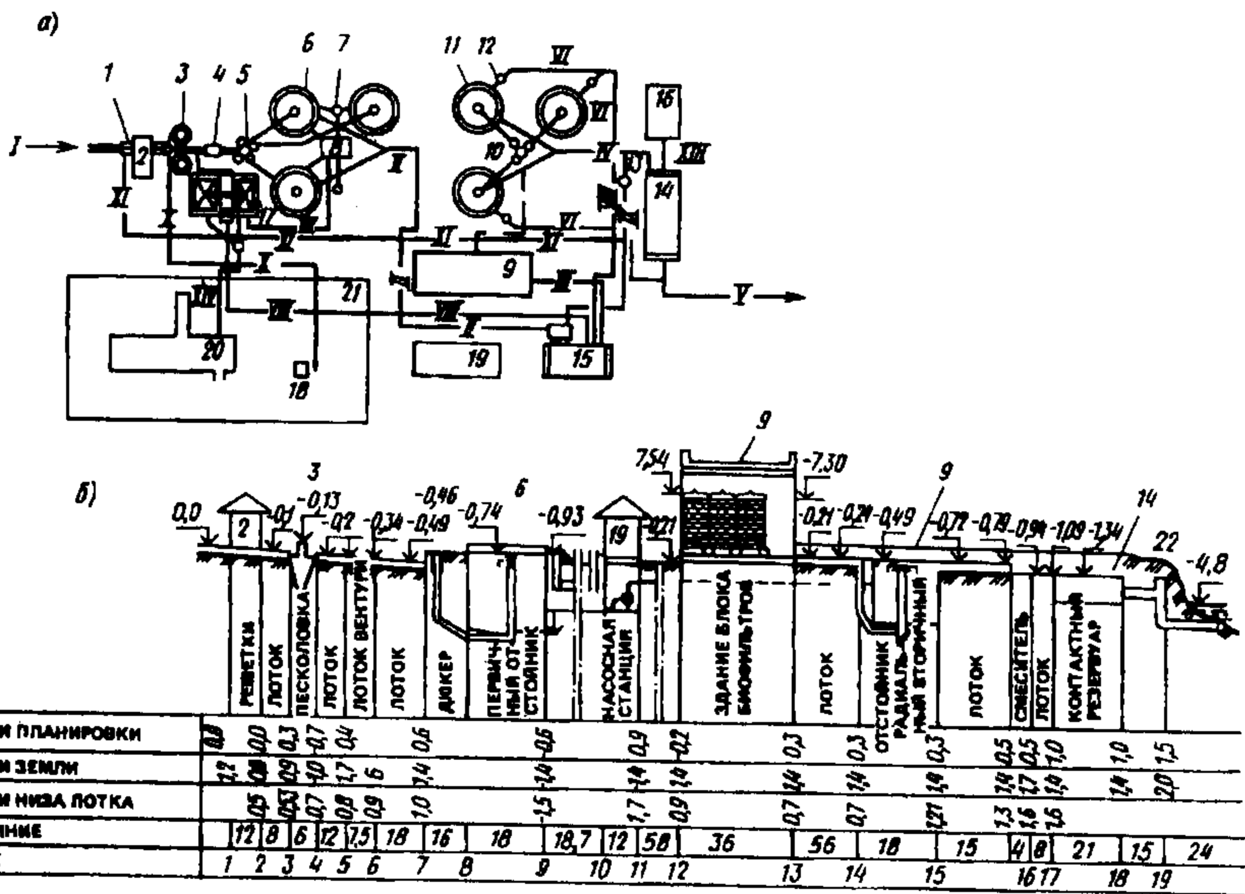
Рис. 12.21. Технологическая схема станции биофильтрации пропускной способностью 25 тыс.м 3 /сут (а) и высотная схема движения сточной воды по очистным сооружениям (б):
