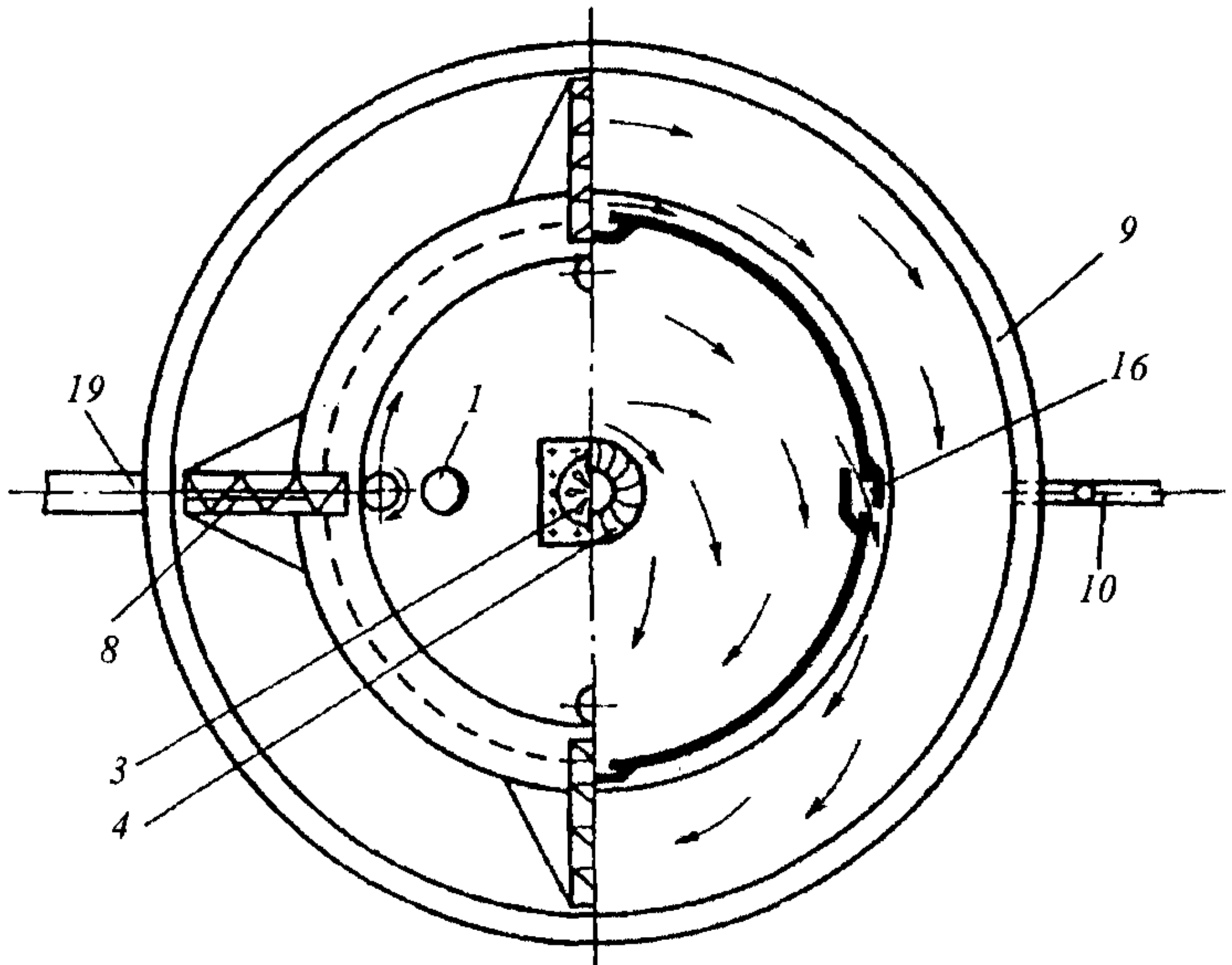
Рис. 11.23. Окситенк:
