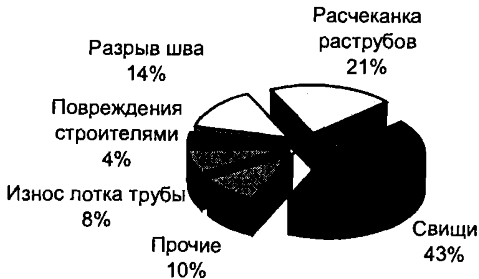
Рис. 21.2. Основные причины отказов напорных трубопроводов
