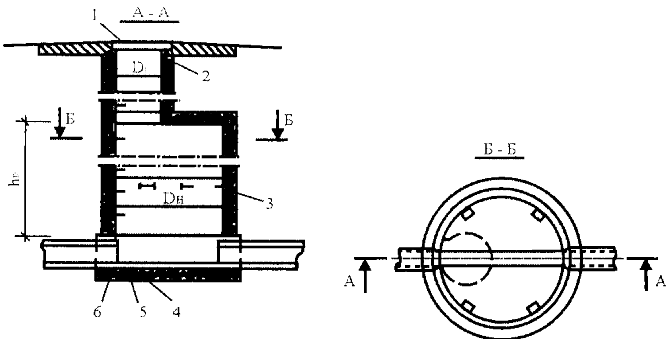
Рис. 6.6. Смотровой колодец:
