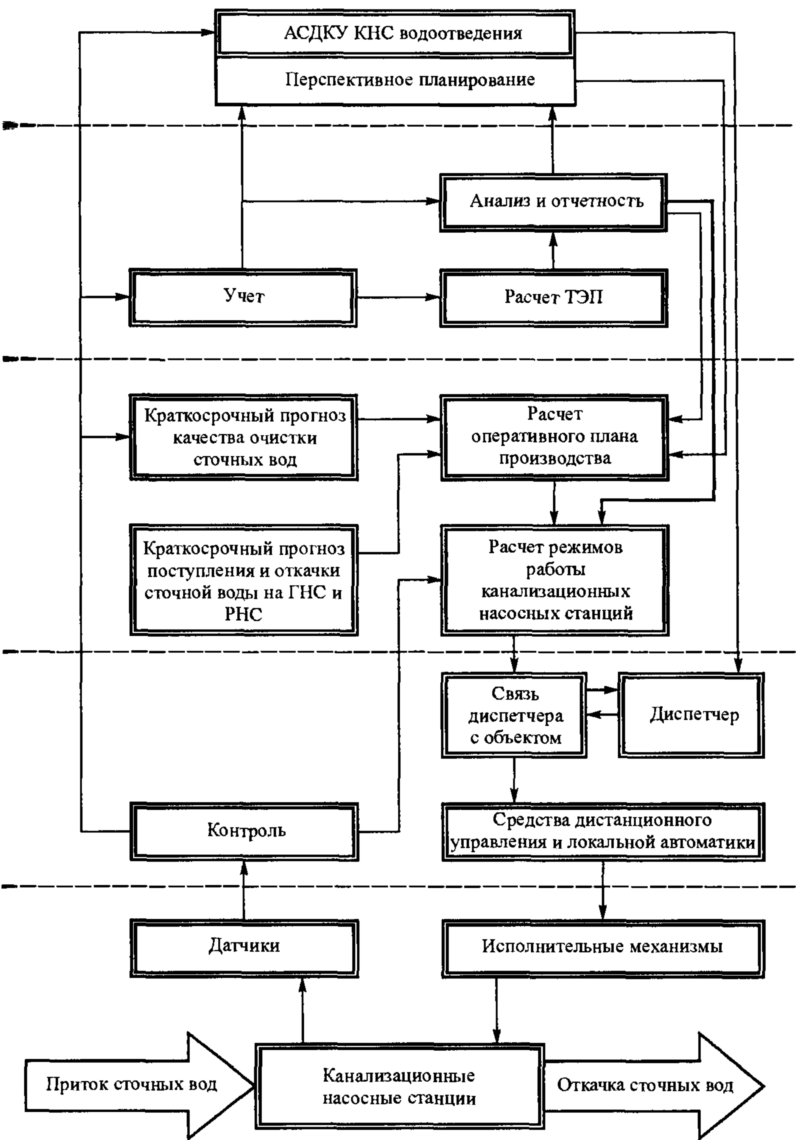
Рис. 20.2. Функциональная структура АСУ насосными станциями
