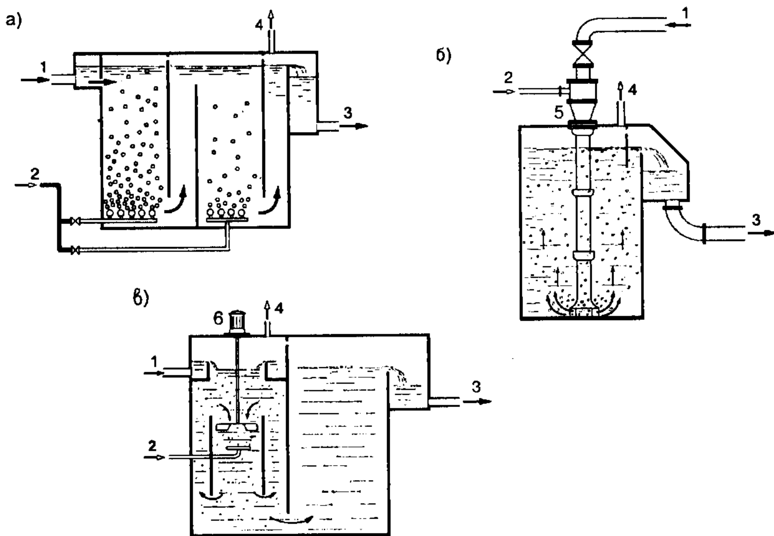
Рис. 13.10. Контактные камеры:
