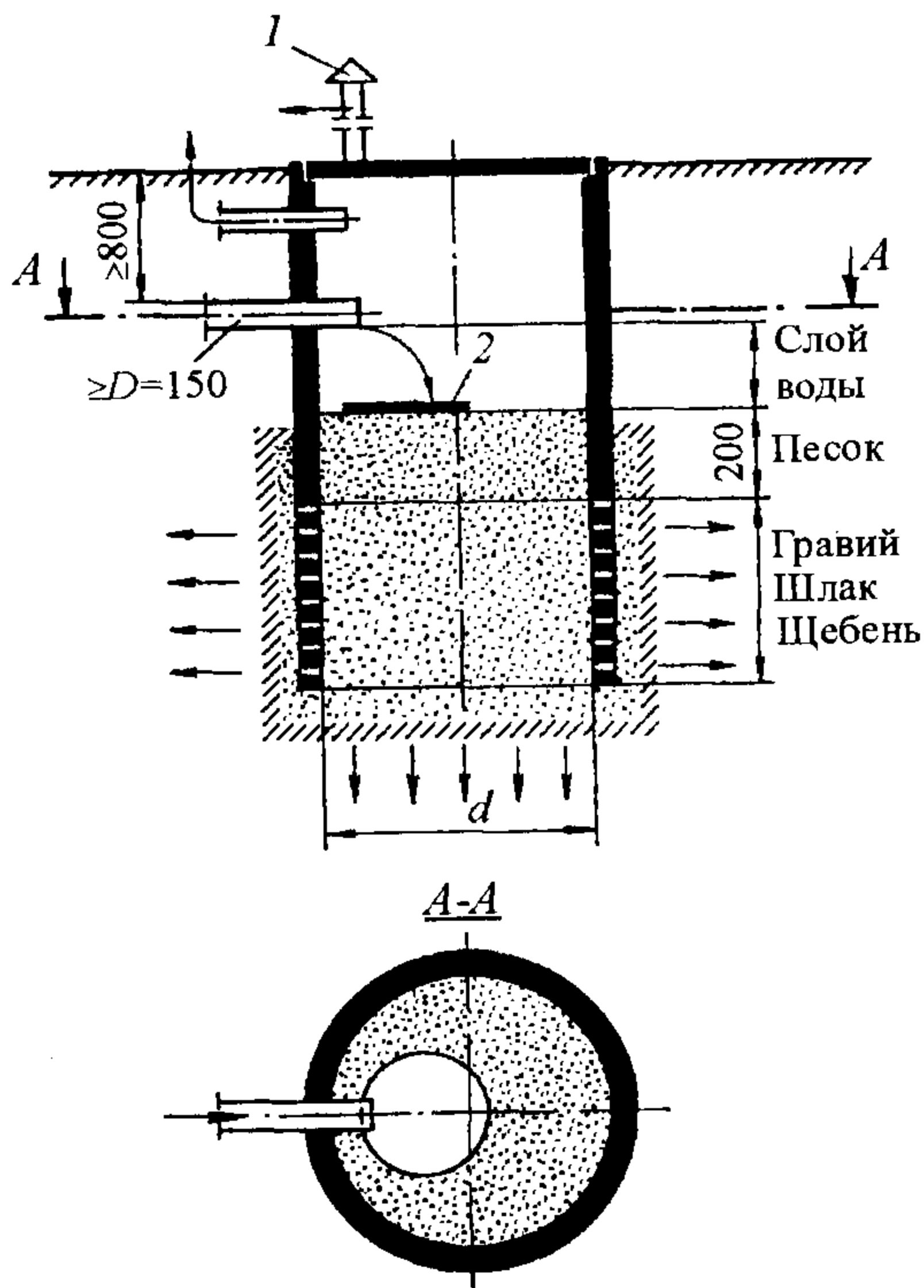
Рис. 24.2. Фильтрующий колодец:
