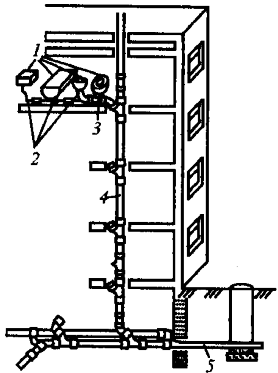
Рис. 1.2. Схема внутренней водоотводящей системы жилого дома:
