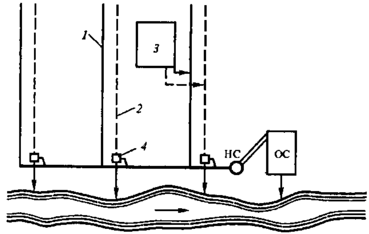
Рис. 1.6. Схема полураздельной системы водоотведения:
