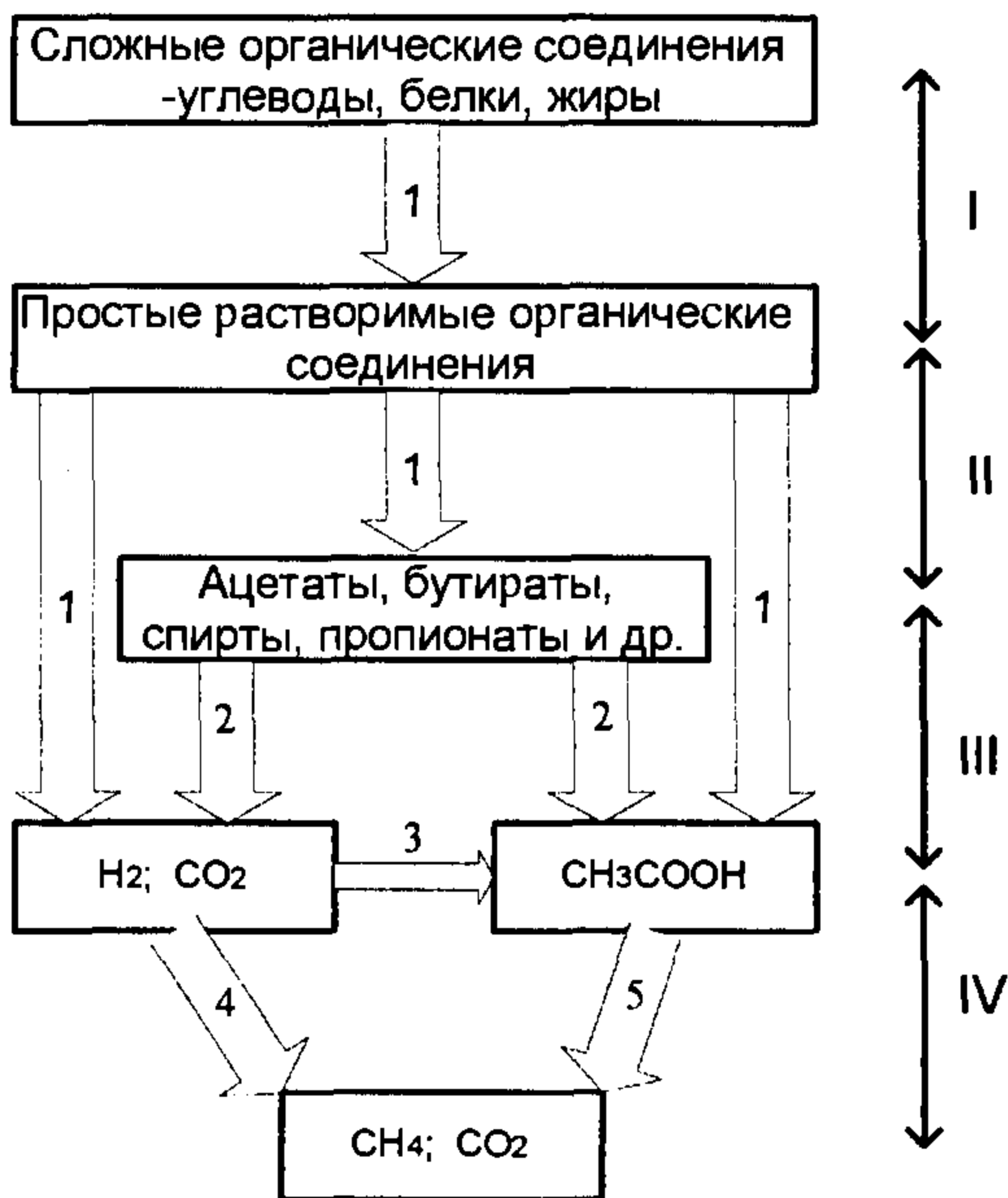
Рис. 15.11. Схема анаэробного метанового сбраживания осадков:
