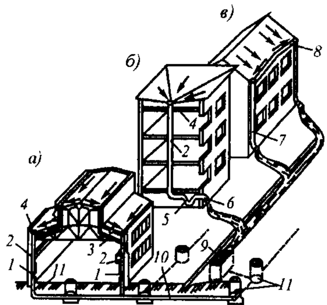
Рис. 1.3. Схемы внутренних водостоков:
