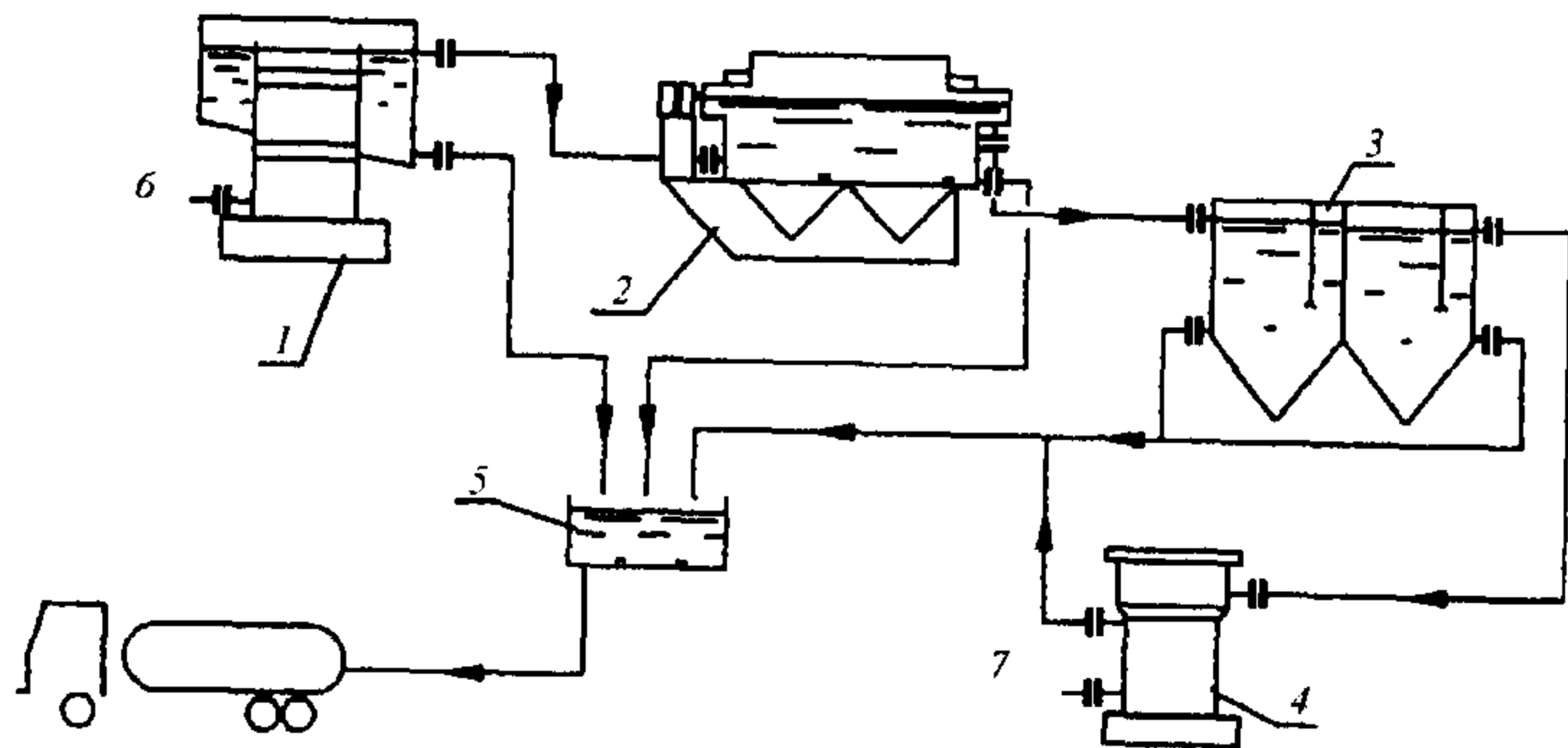
Рис. 23.10. Комплекс локальной очистки производственных сточных вод:
