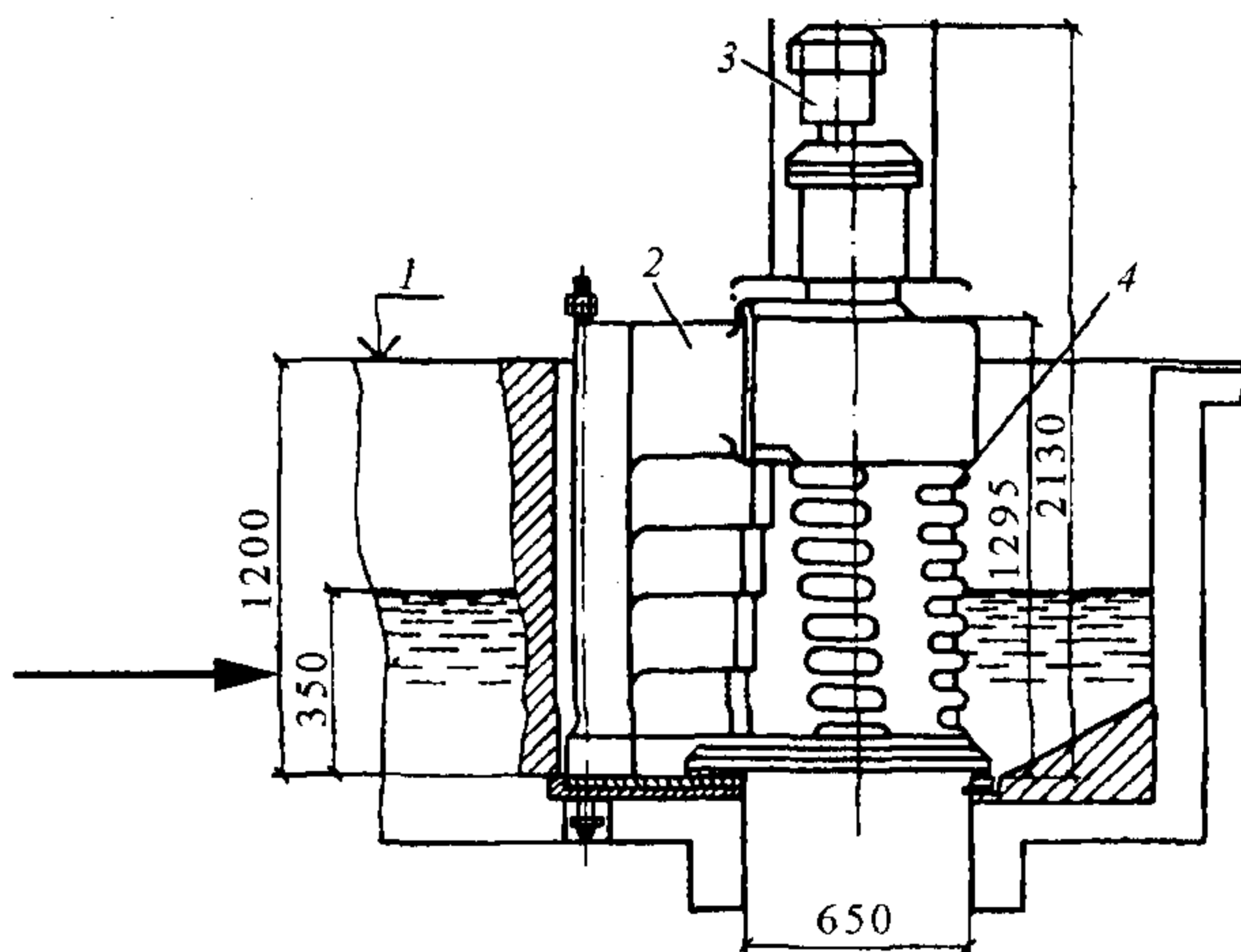
Рис. 7.2. Решетка-дробилка РД-600:
