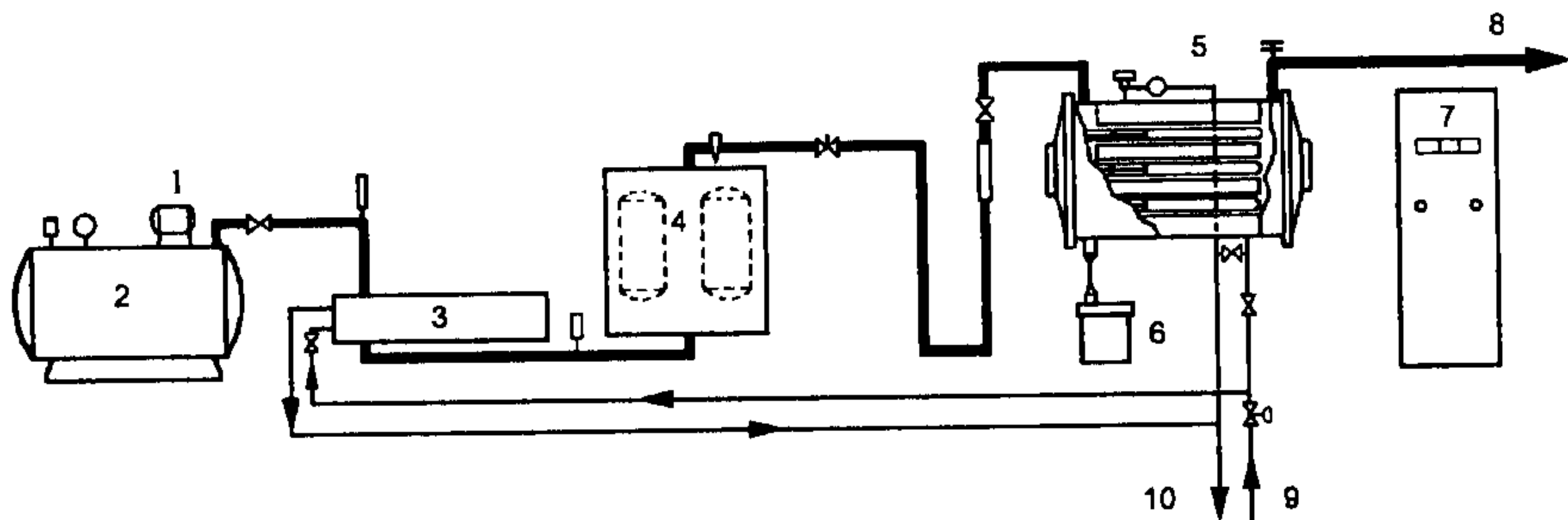
Рис. 13.9. Схема установки получения озона:
