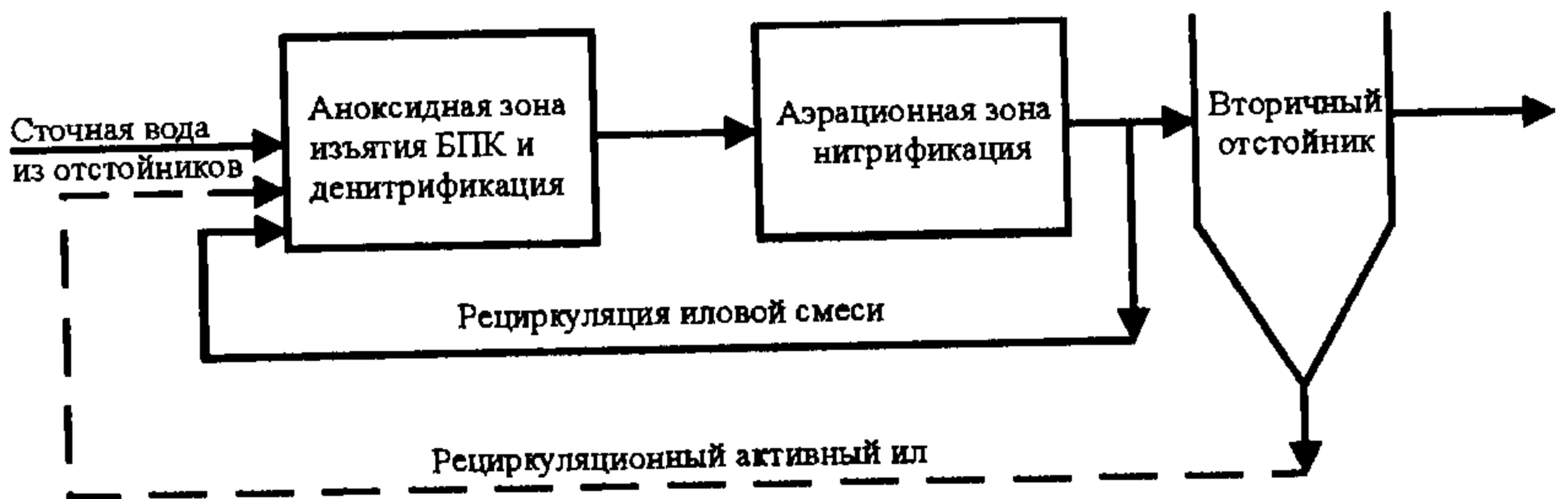
Рис. 11.30. Схема работы аэротенка с удалением азота по одноилловой системе
