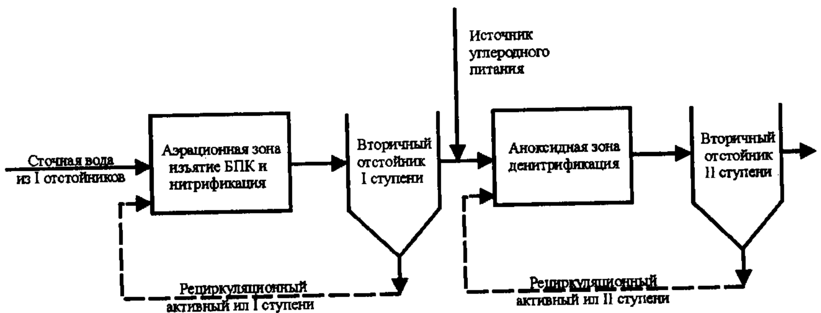
Рис. 11.31. Схема работы аэротенка с удалением азота по двухилловой системе
