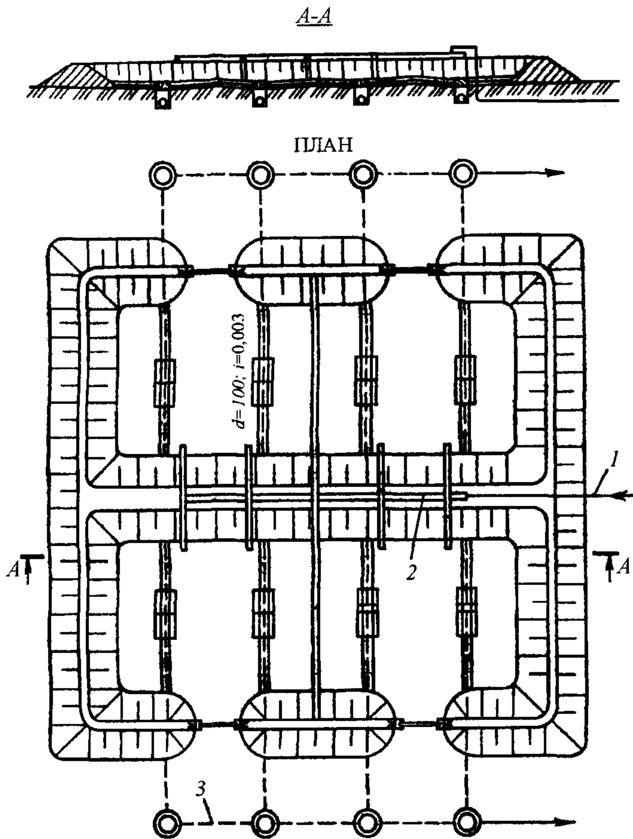
Рис. 16.1. Песковая площадка:
