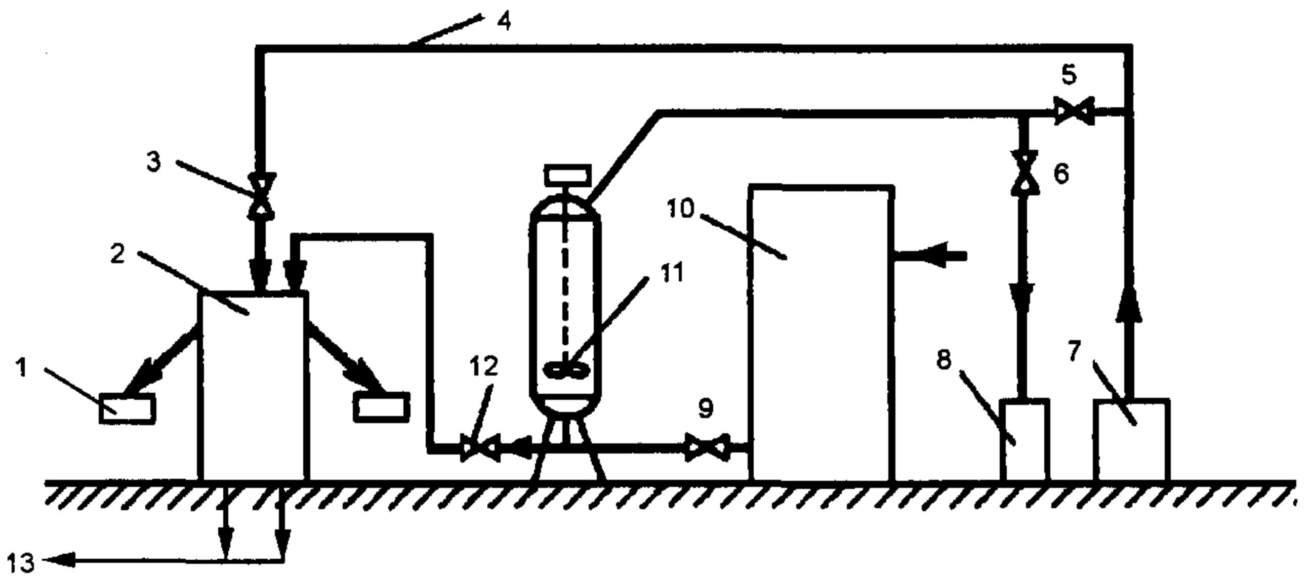
Рис. 16.12. Технологическая схема фильтр-прессования осадков:
