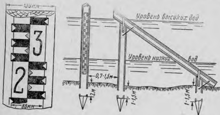
Рис. 2. Водомерная рейка.
